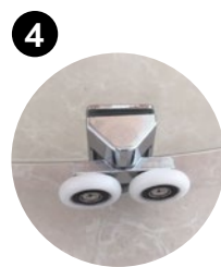
4 Rugós kivitelű alsó görgők Mekkönnyíti a kabin tisztítását mert könnyen kimozdítható az ajtó.
